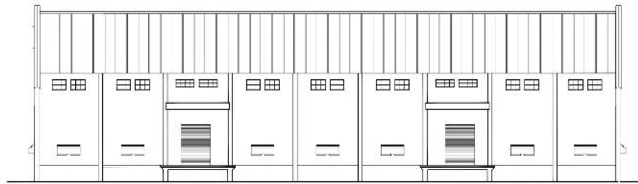
ELEVATION
